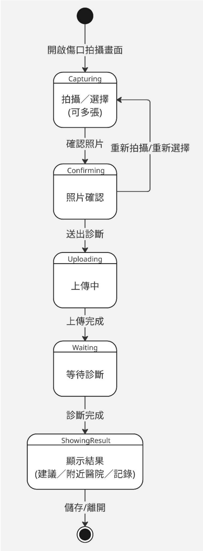
圖 7-4-2 傷口拍攝狀態機
