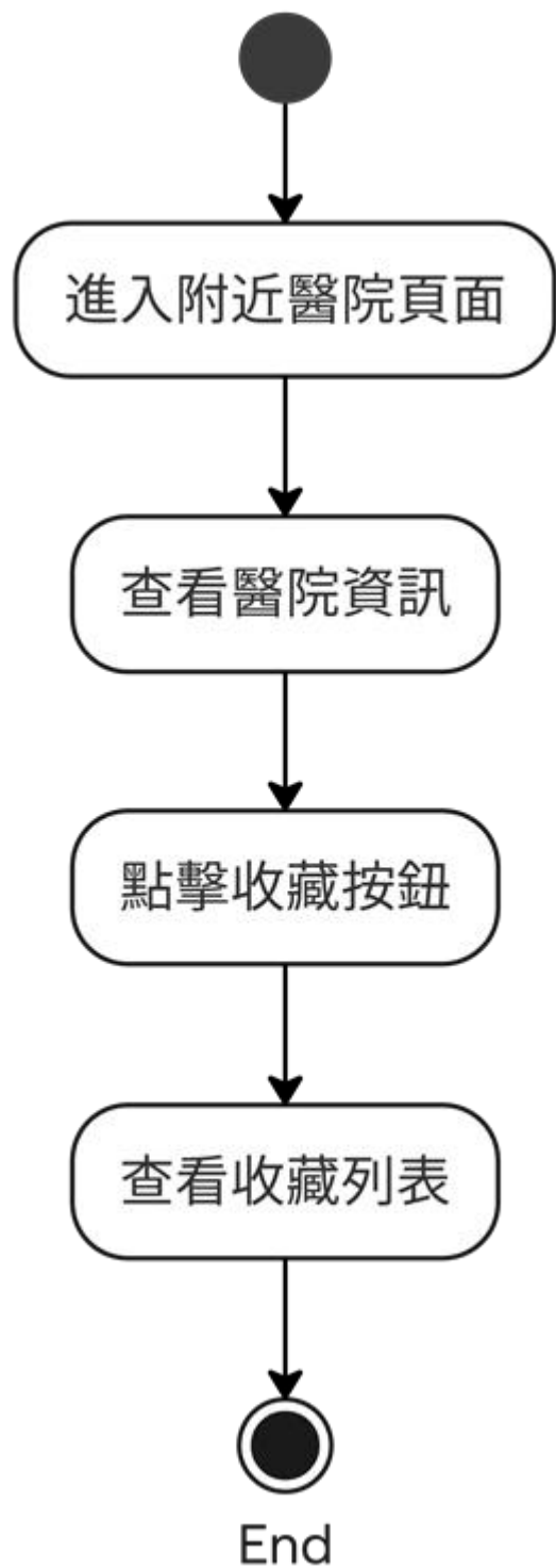
圖 5-3-6 收藏醫院活動圖
