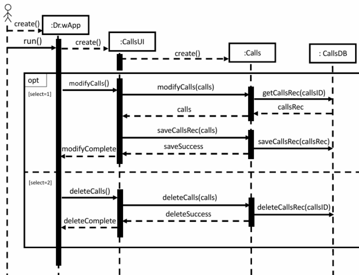
圖 6-1-3 管理護理提醒循序圖
