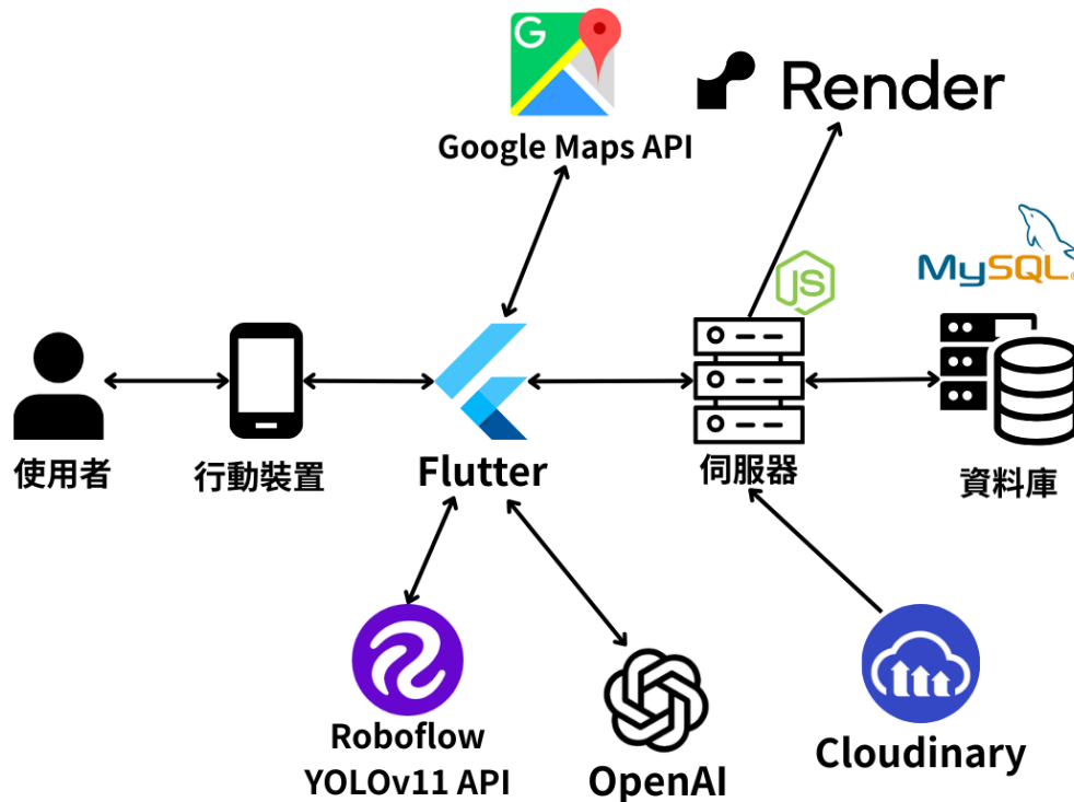
圖 3-1-1 系統架構-圖示
