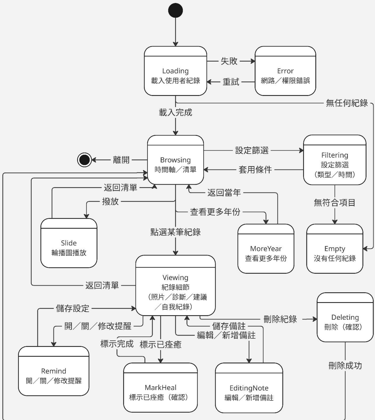
圖 7-4-4 紀錄冊瀏覽與管理狀態機
