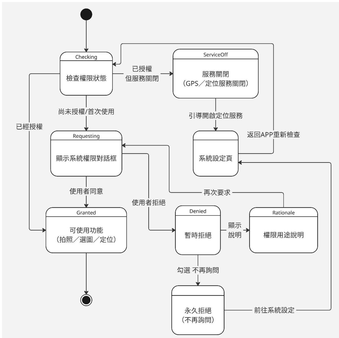
圖 7-4-5 檢查權限狀態機
