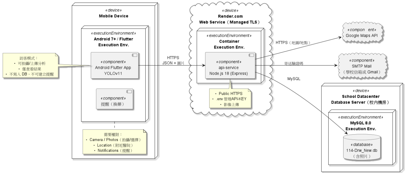
圖 7-1-1 佈署圖
