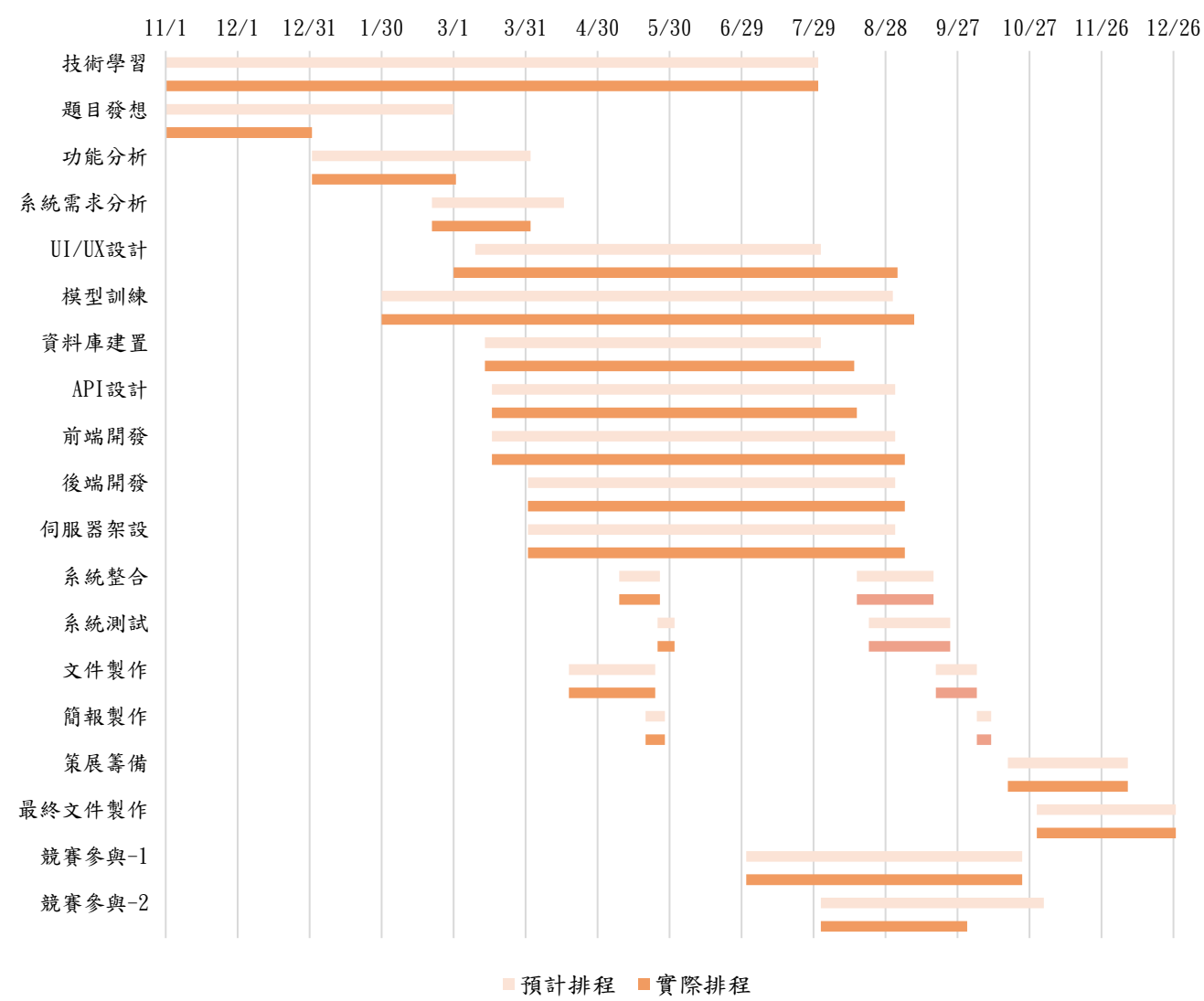
圖 4-1-1 甘特圖
