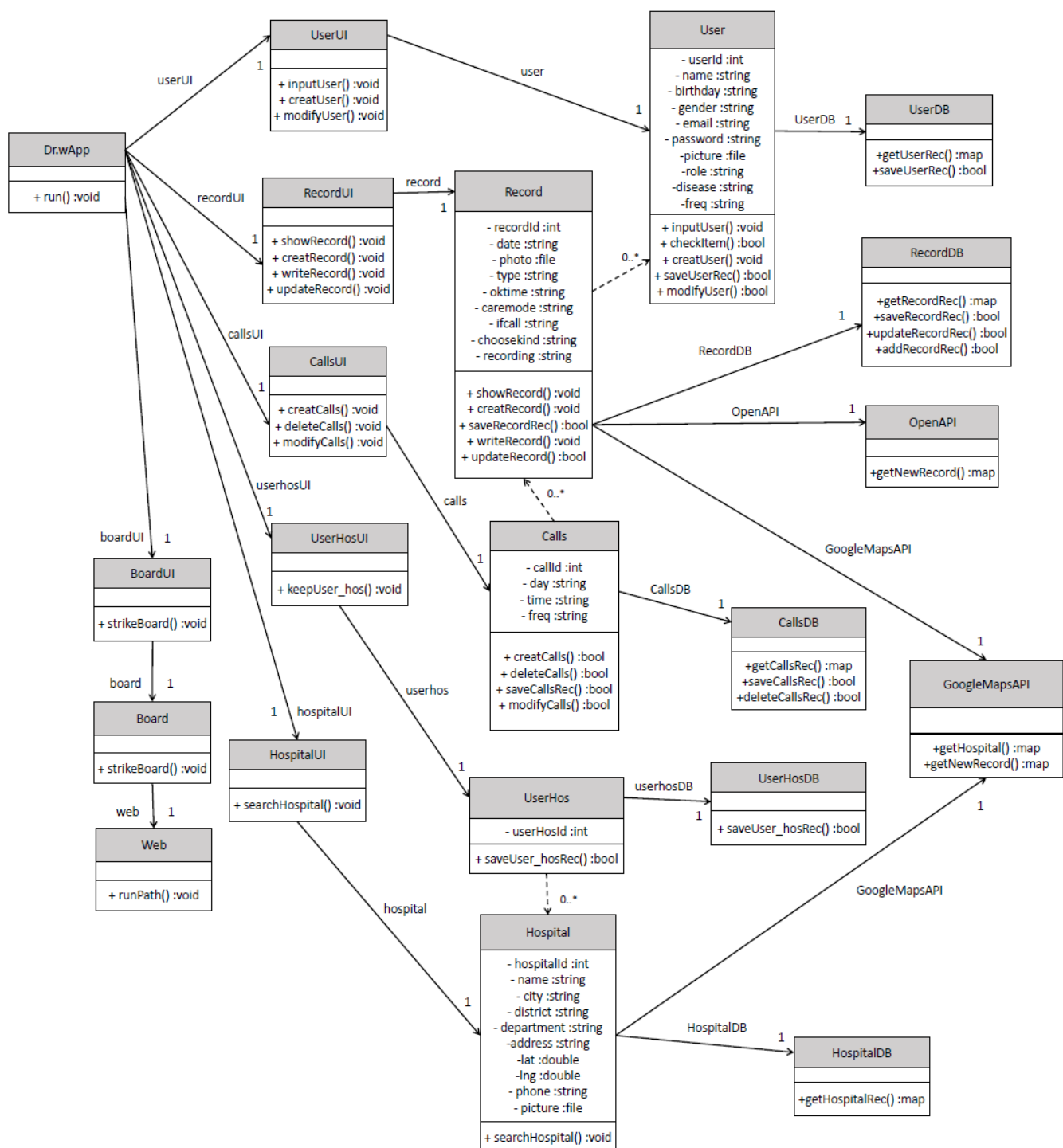
圖 6-2-1 設計類別圖
