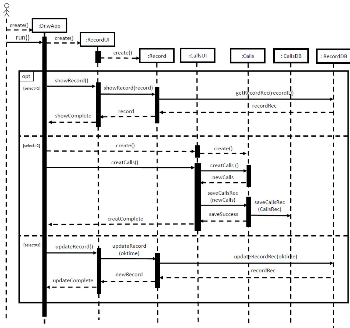
圖 6-1-6 查看紀錄簿循序圖
