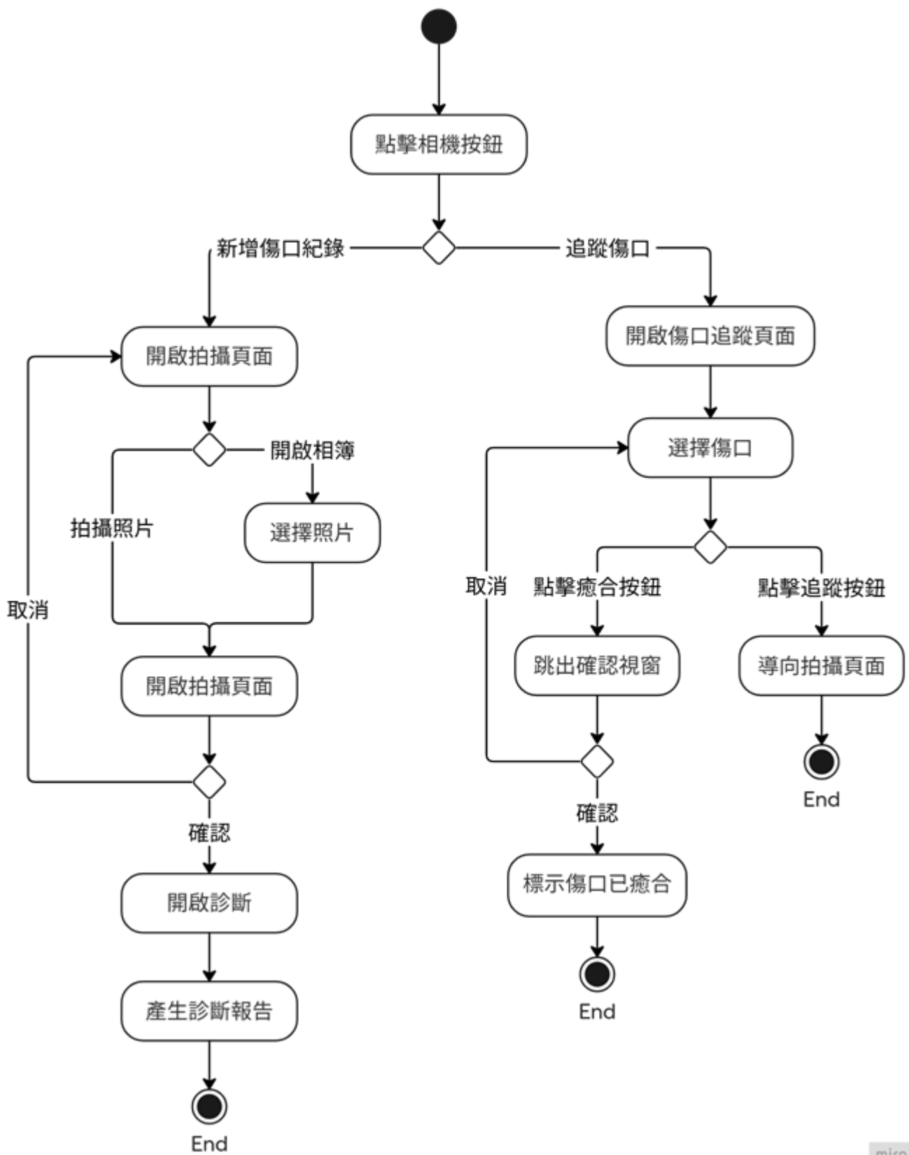
圖 5-3-8 上傳照片活動圖
