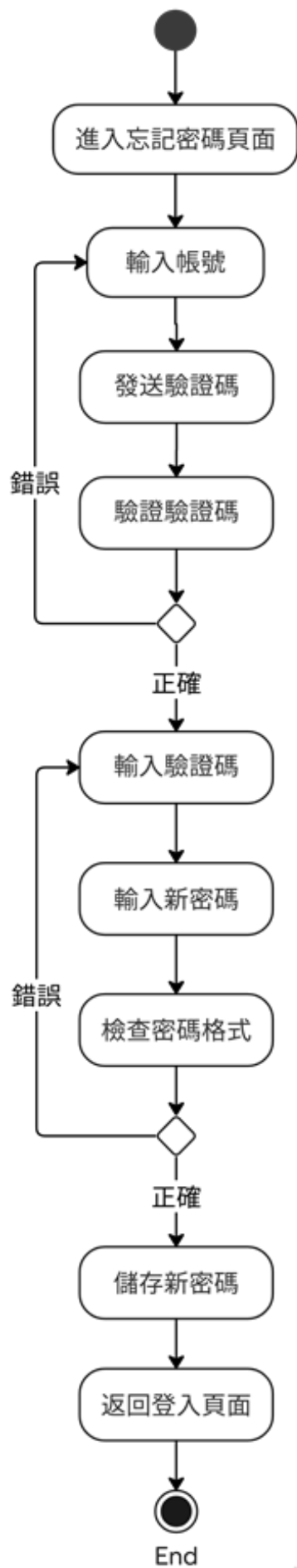
圖 5-3-3 忘記密碼活動圖
