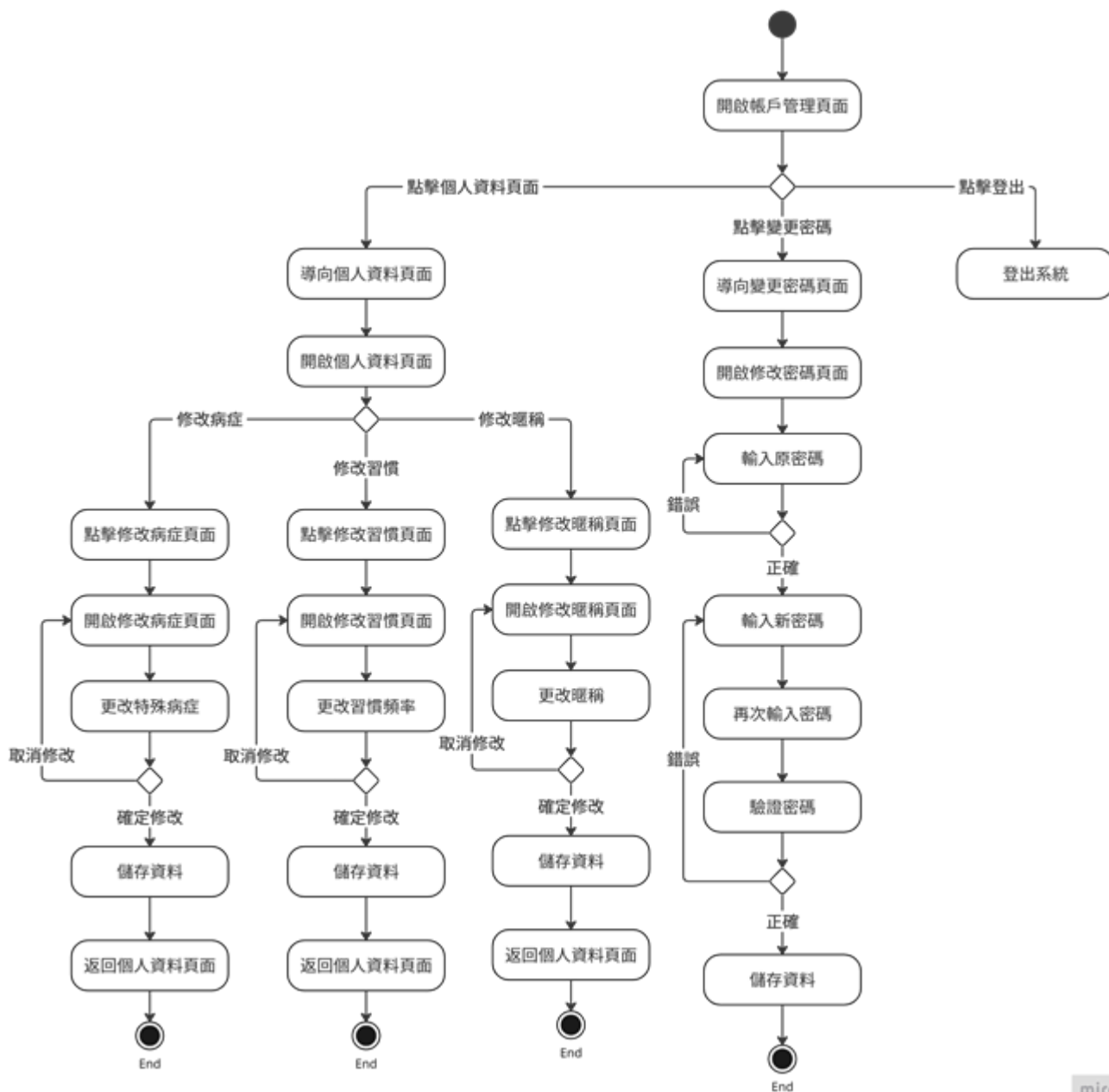
圖 5-3-10 管理帳戶活動圖
