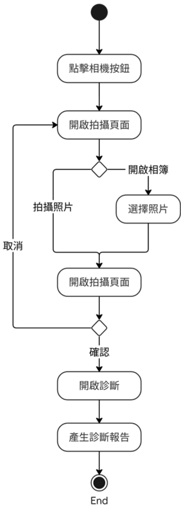
圖 5-3-12 上傳照片(訪客)活動圖
