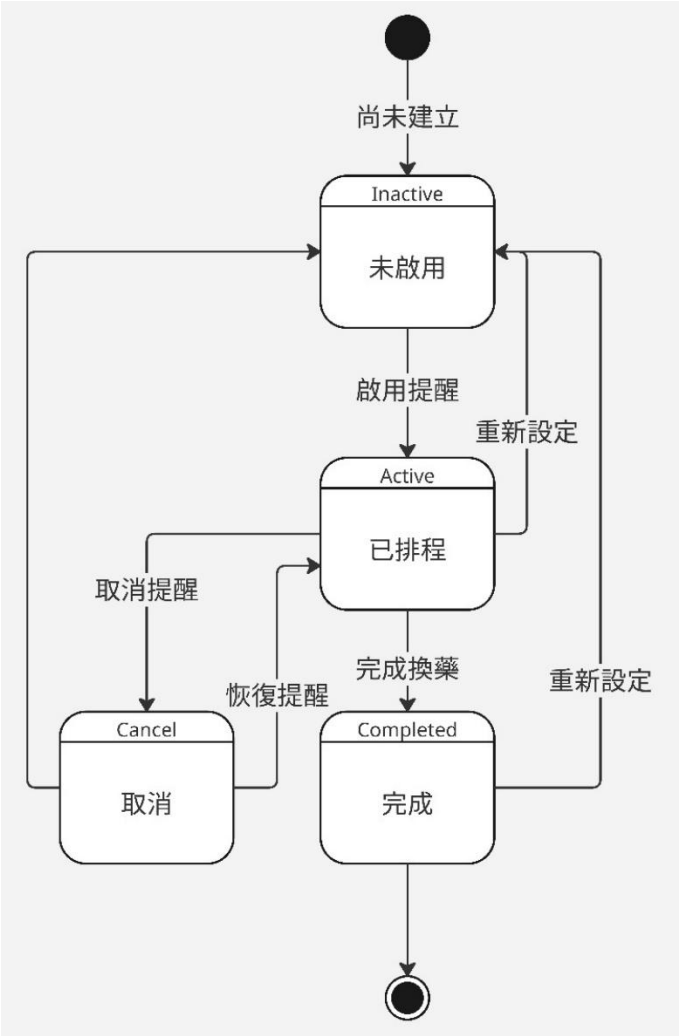
圖 7-4-1 換藥提醒狀態機
