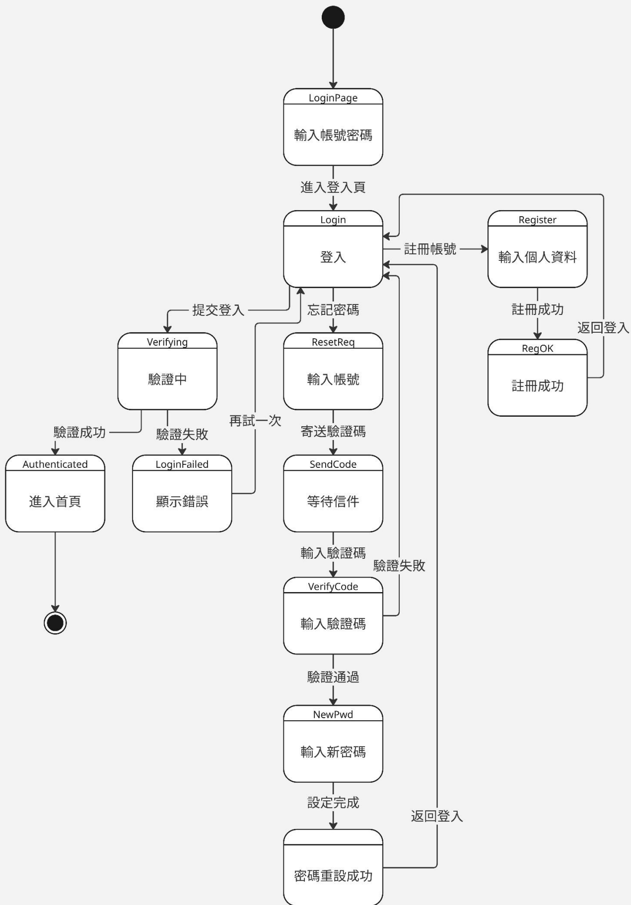
圖 7-4-3 帳號流程狀態機
