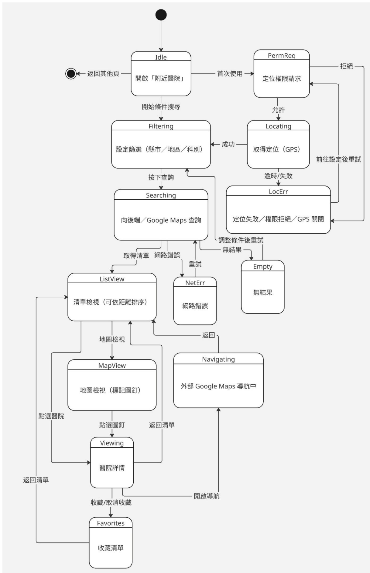
圖 7-4-6 醫院搜尋與導航狀態機
