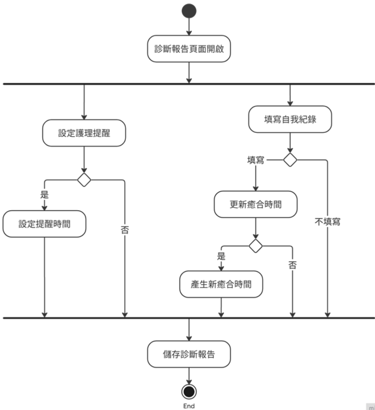
圖 5-3-11 查看診斷報告活動圖
