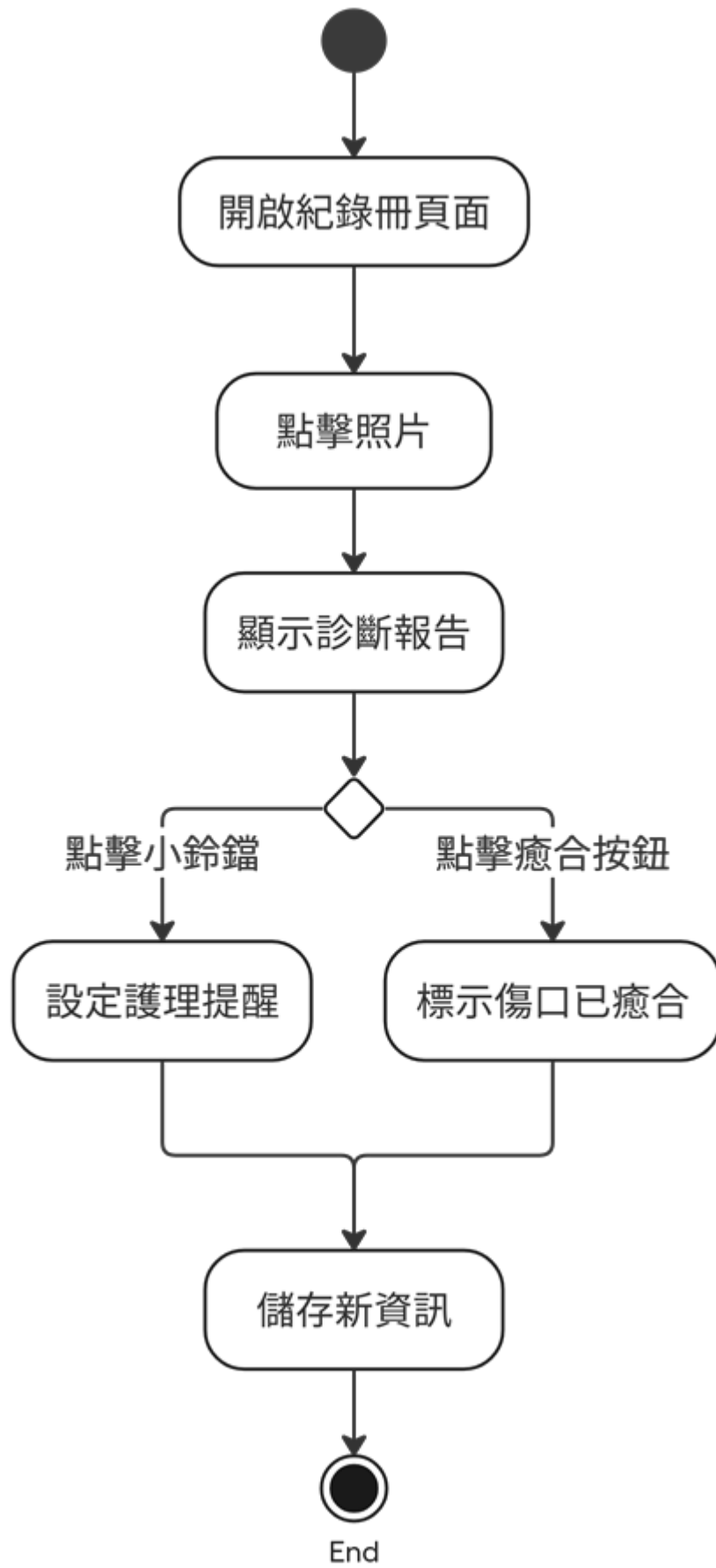
圖 5-3-9 查看紀錄簿活動圖
