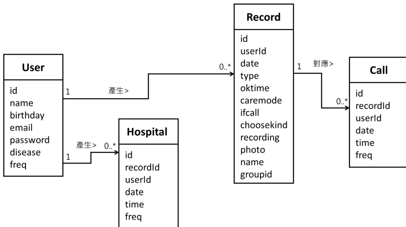
圖 5-4-1 分析類別圖
