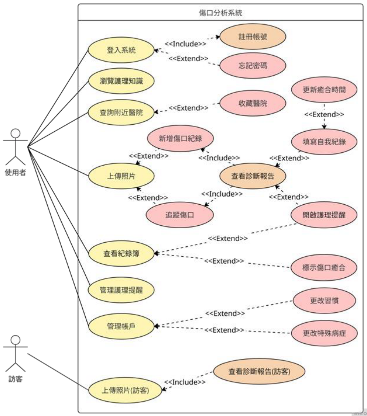
圖 5-2-1 使用個案圖
