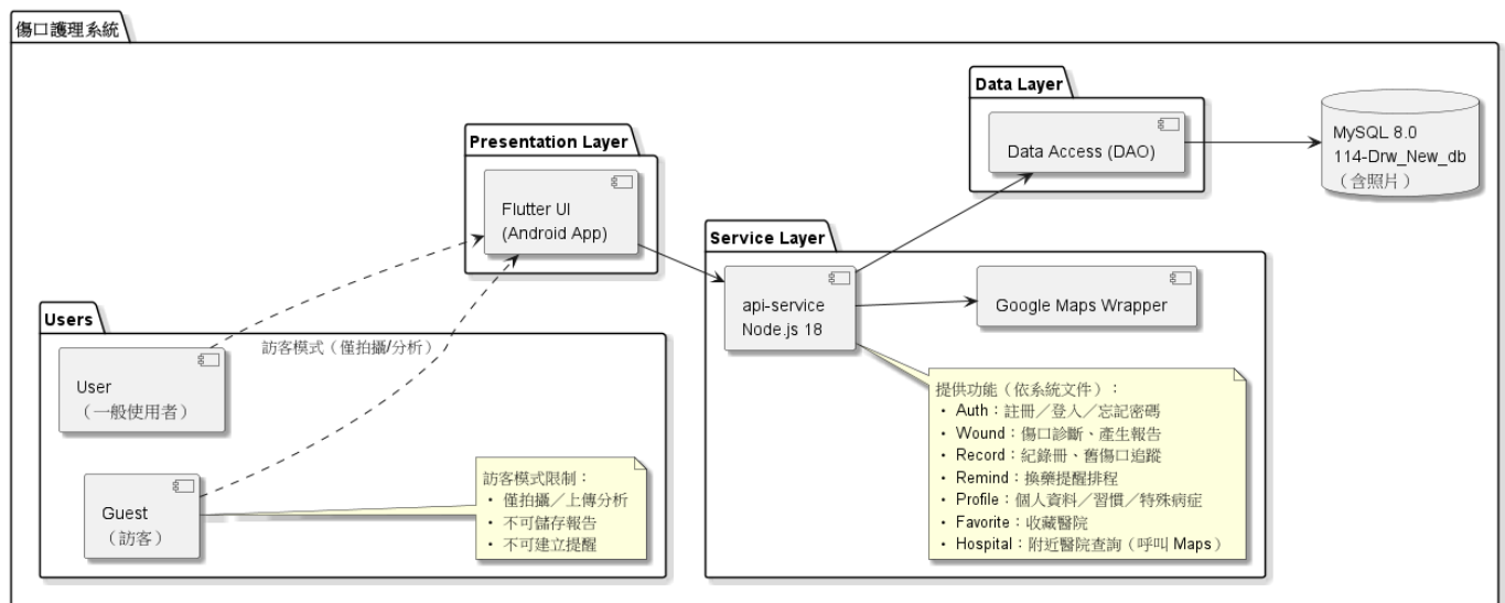
圖 7-2-1 套件圖
