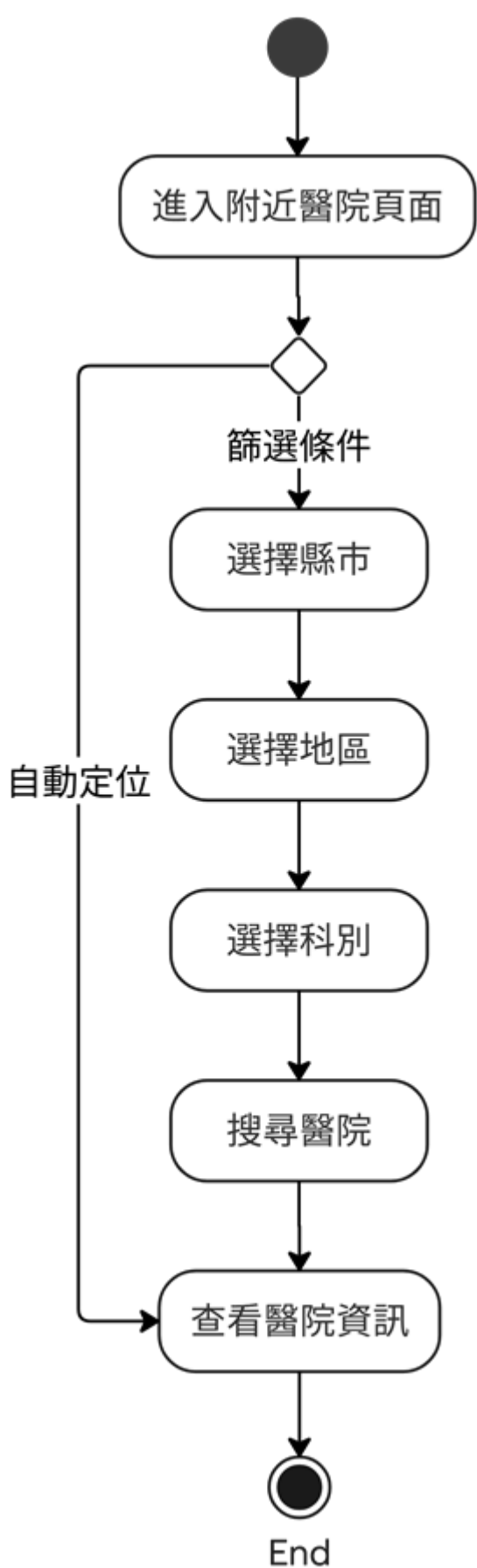
圖 5-3-5 查詢附近醫院活動圖
